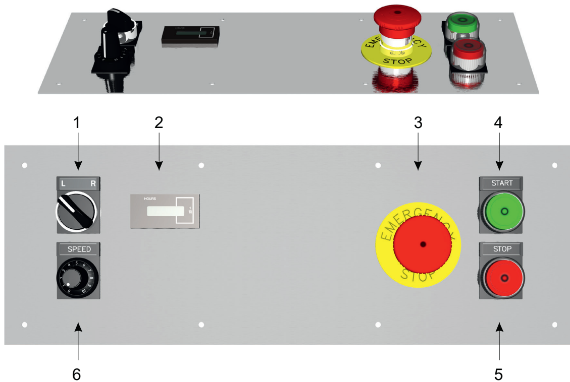
Figur 4.2 SC-650 kontrollpanel
