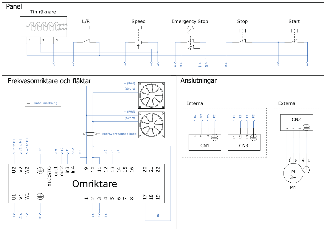
Figur 61 Elschema SC-650
